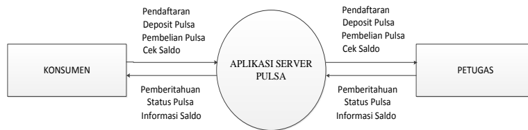
Gambar 1. Diagram Konteks
